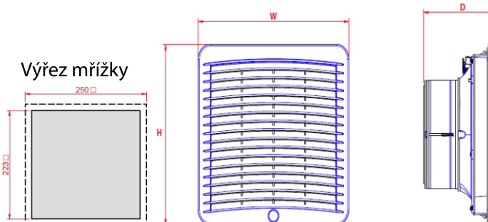
Ventilátory s filtrem
