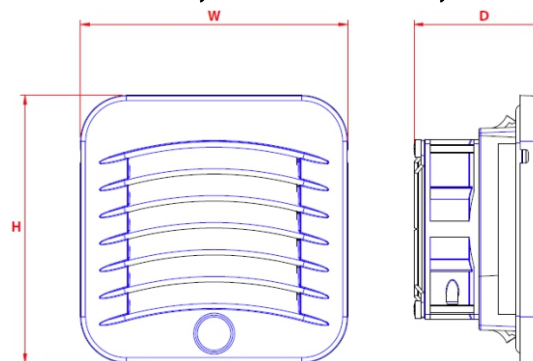
Rozměry ventilátoru a mřížky
