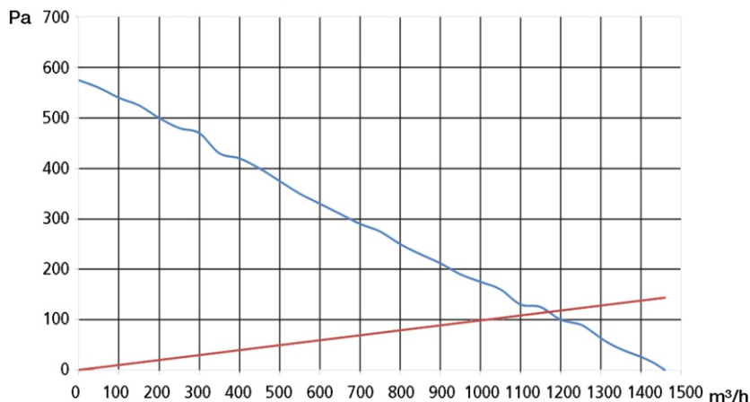
Graf výkonu ventilátorů TB 250
