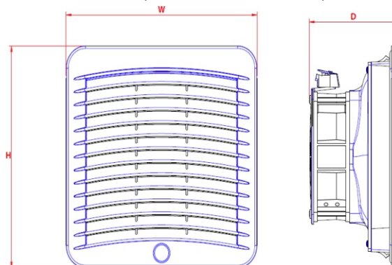
Rozměry ventilátoru a mřížky
