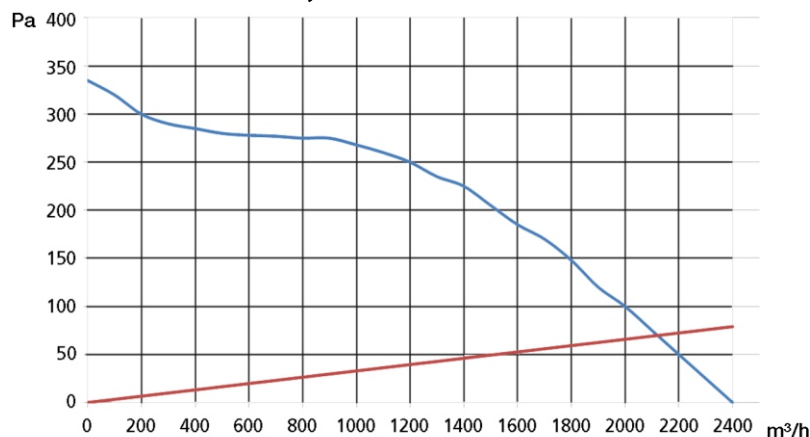
Graf výkonu ventilátorů TB 350
