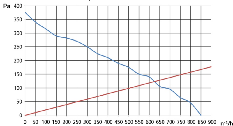
Graf výkonu ventilátorů TB 220
