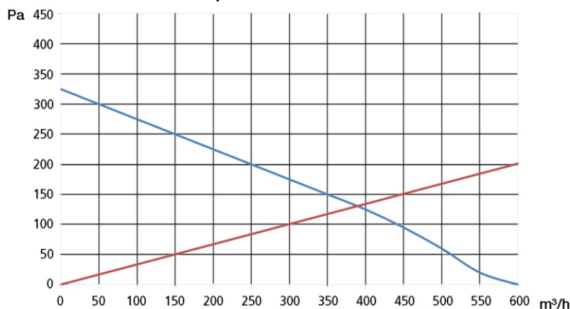
Graf výkonu ventilátorů TB 190
