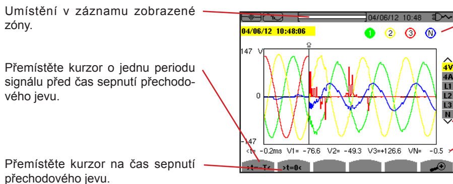
Obrázek 41: Příklad zobrazení přechodových jevů v 5vodičové třífázové soustavě v podobě křivek
