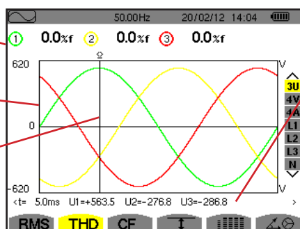
Obrázek 67: Obrazovka 3U THD
