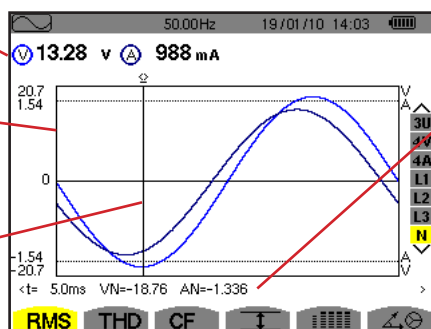
Obrázek 66: Obrazovka RMS pro nulový vodič
