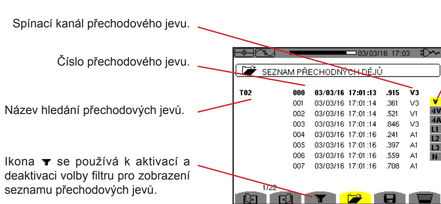
Obrázek 40: Obrazovka seznamu přechodových jevů pro 5vodičovou třífázovou soustavu
