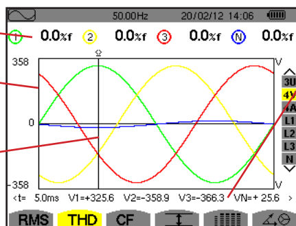
Obrázek 68: Obrazovka 4V THD
