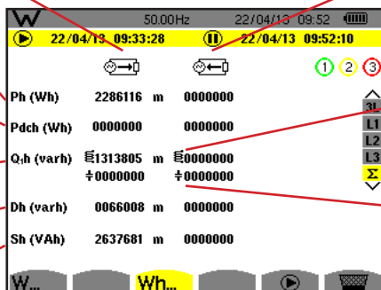
Obrázek 116: Obrazovka celkových energií spotřebovaných a generovaných v Σ
