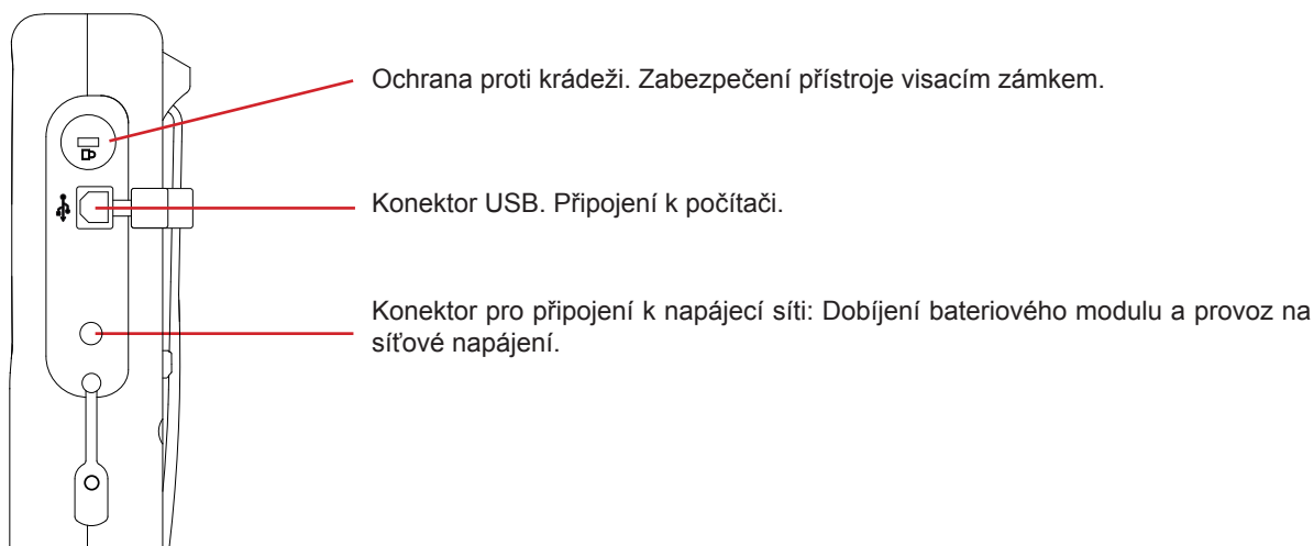
Obrázek 4: Boční konektory
