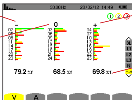
Obrázek 60: Obrazovka expertního režimu napětí mezi fází a nulovým vodičem (třífázové soustavy s nulovým vodičem)
