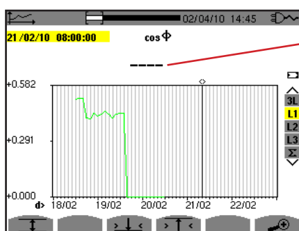
Obrázek 106: \cos \Phi (L1) ukončení zavádění/výpočtu hodnot
