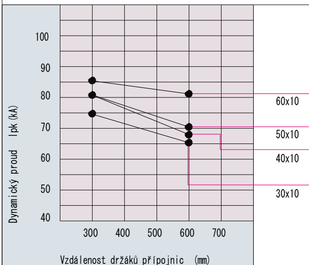
Držák přípojnic č. 01479.000 systém 100Energy
