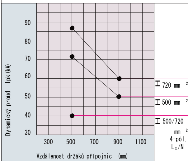
Držák přípojnic č. 01231.000 / 01116.000, 3 a 4-pól systém 60Classic 1250 A / 1600 A
