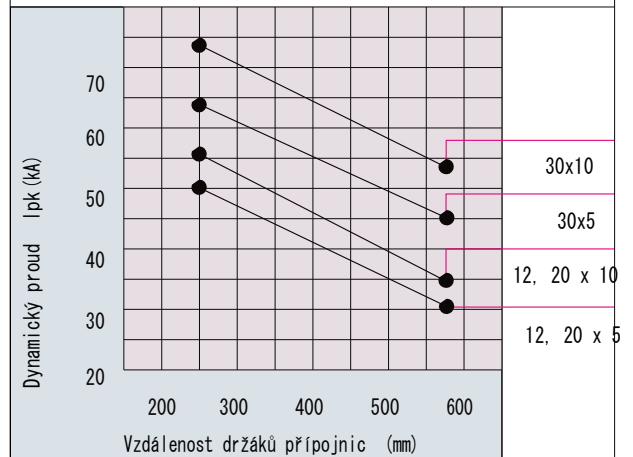
Držák přípojnic č. 01495.000 / 01500.000 / 01315.000 / 01316.000 systém 60Classic
