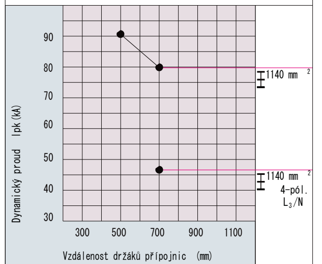
Držák přípojnic č. 01742.000 systém 185Power
