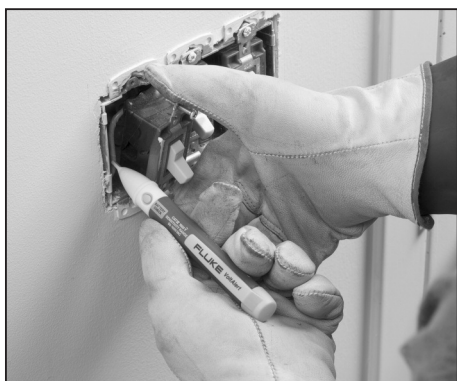
Fluke 2 AC VoltAlert
